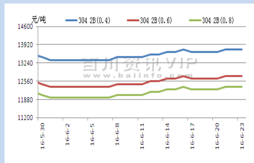
无锡联众 201/NO.1 平板走势图
