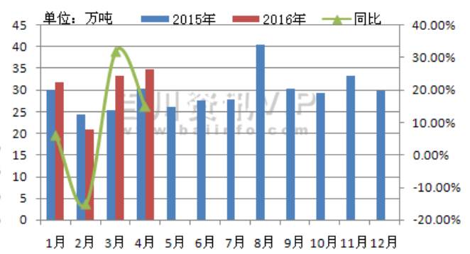
2016年国内不锈钢出口量走势图
