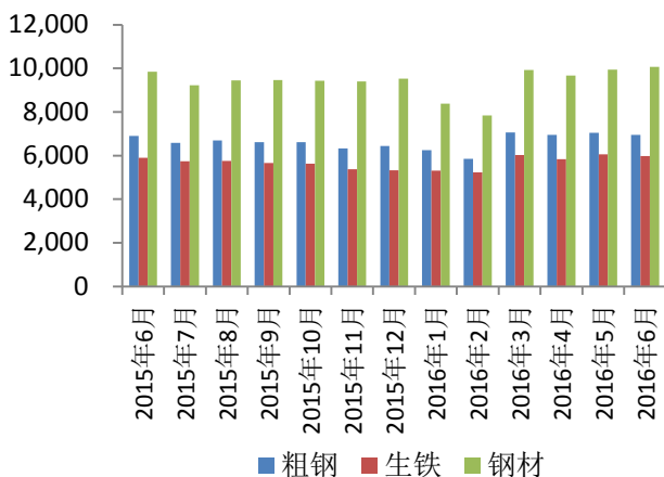
图 51: 国内粗钢、生铁、钢材产量走势 (万吨)
