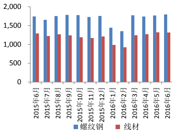
图 52: 国内螺纹钢线材产量走势 (万吨)
