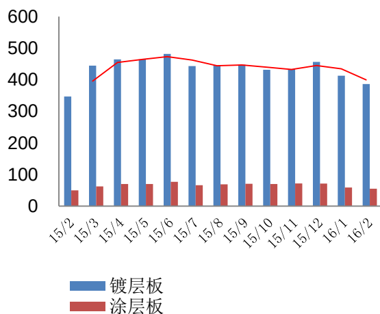
图 55: 国内涂镀产量走势 (万吨)
