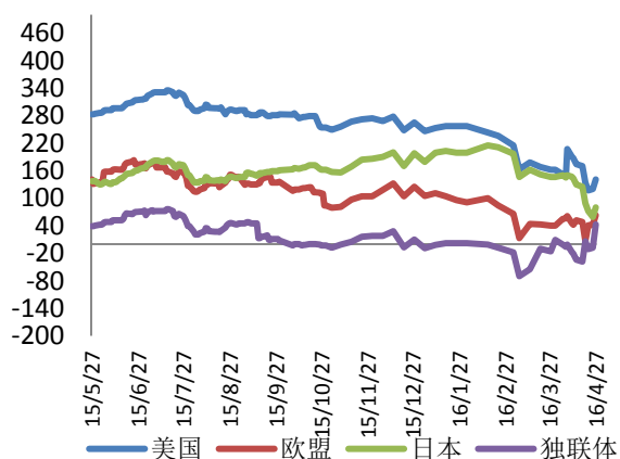
图 23：螺纹钢国际国内价差走势（美元/吨）
