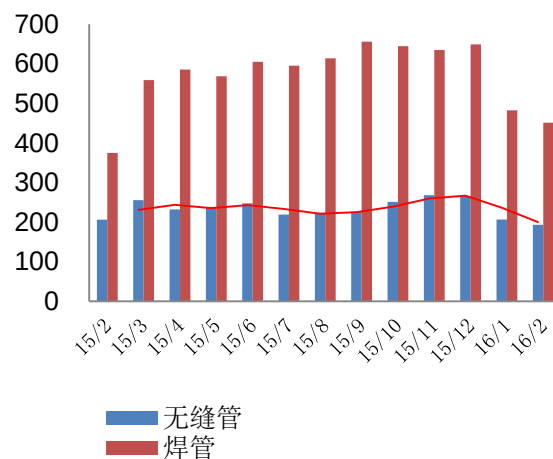
图 56: 国内管材产量走势 (万吨)
