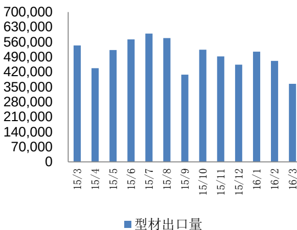
图 62：国内型材出口量走势（吨）
