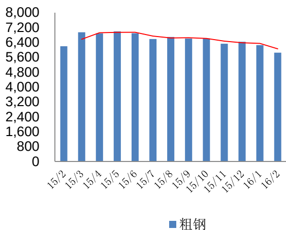
图 51: 国内粗钢产量走势 (万吨)
