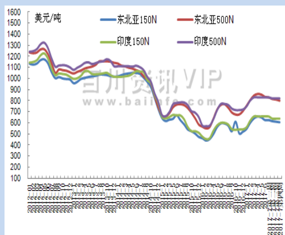
国际 II 类基础油到岸价平均价格走势
